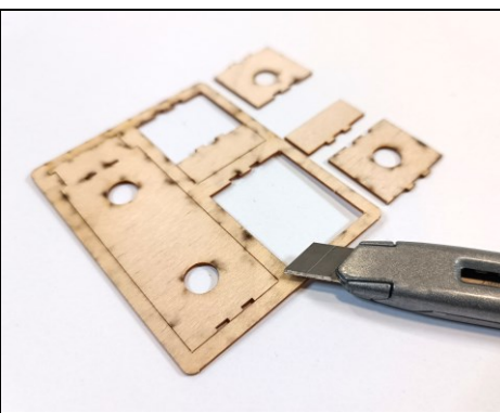
Die kleine Stege an der Unterseite durchtrennen.
