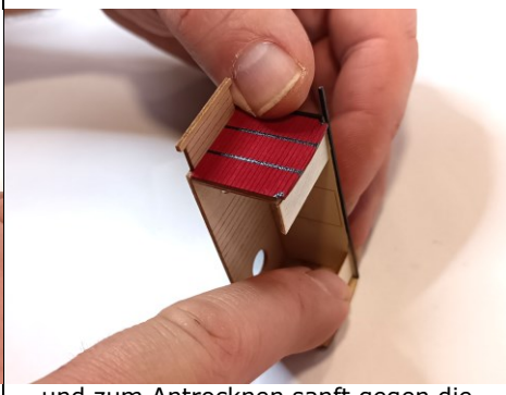
und zum Antrocknen sanft gegen die Unterlage ddrücken.
