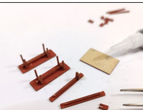
Erst Längsträger aufkleben, dann Beine montieren.
