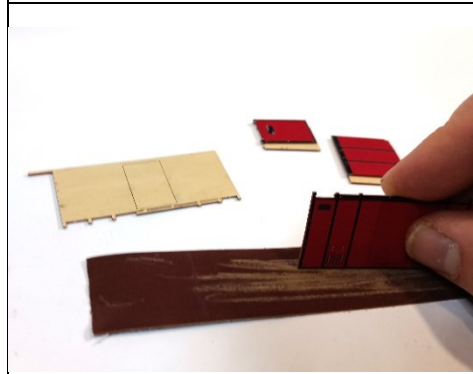
Die Reste der Stege wegschleifen.
