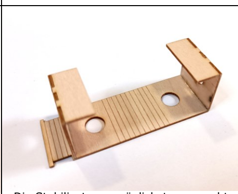
Die Stabilisatoren möglichst waagrecht ankleben.
