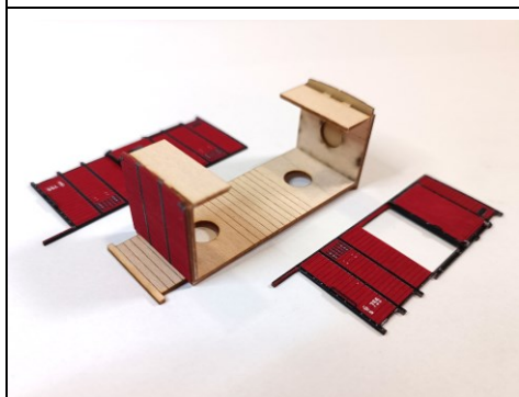
Die Montage der Wagenseiten sollte sorgfältig erfolgen.
